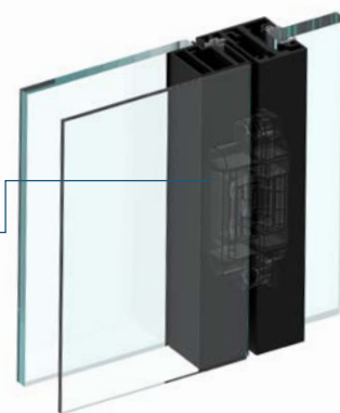
Hidden hinge
