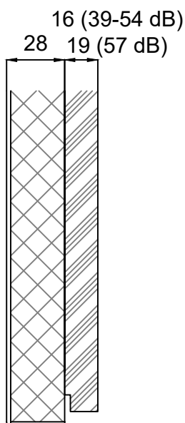
Schnitt A-A section A-A
