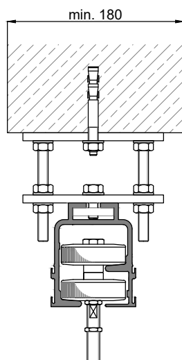
Montage unter Betonsturz Installation on concrete beam
