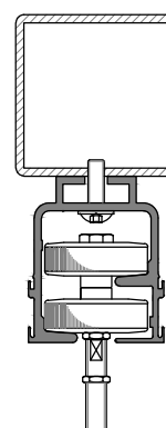
Direktmontage an bauseitigem Vierkantstahl durch Verschrauben direct fixation at square steel profile by screwing
